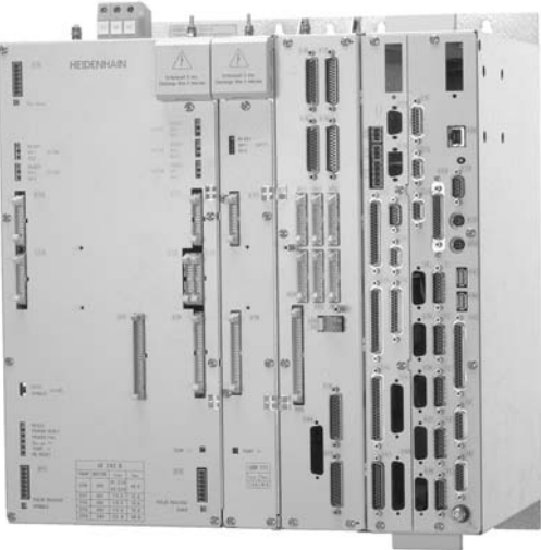
MC 422 B, CC 422 avec variateur compact et module de puissance supplémentaire
