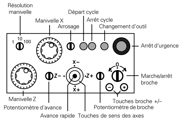
Exemple d'un panneau de commande machine
