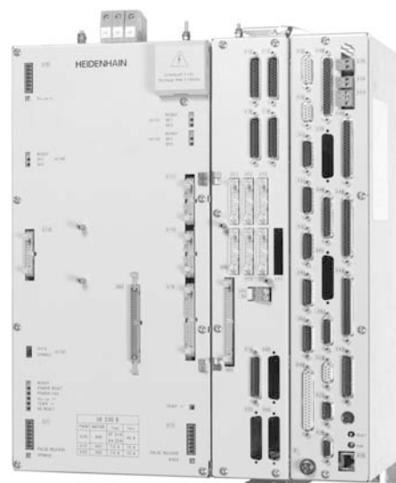
LE 412M avec variateur compact
