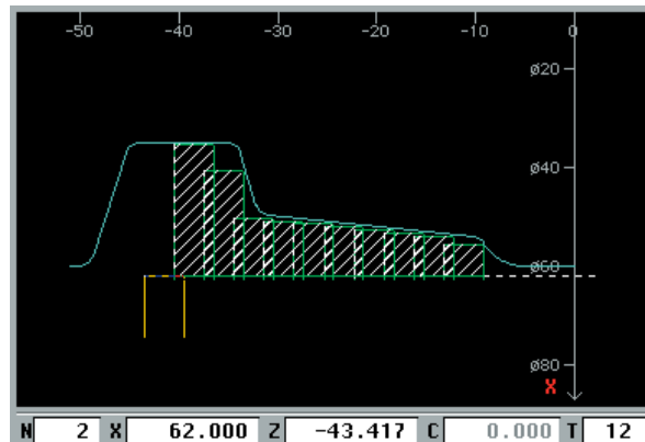
Simulation de la trace de la dent pour vérifier la gorge
