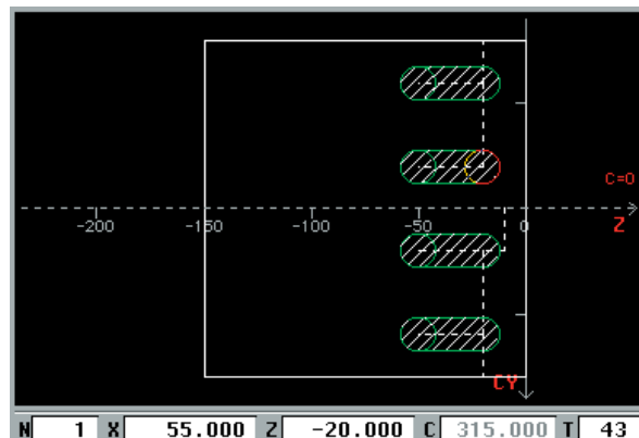
Rainures sur le (déroulé du) pourtour
