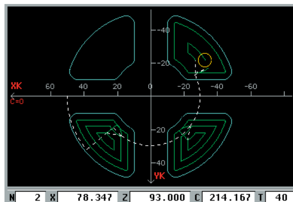
Opération de fraisage sur la face frontale
