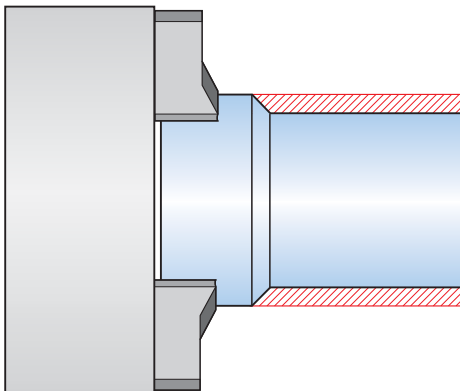
1. Chariotage longitudinal avec chanfrein
