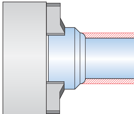
2. Chariotage longitudinal avec rayon
